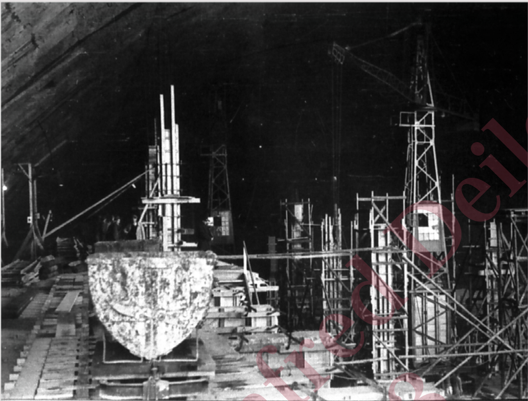
Die Decke im Bereich des Deiches Kahn-FinEnkel wird betoniert.
